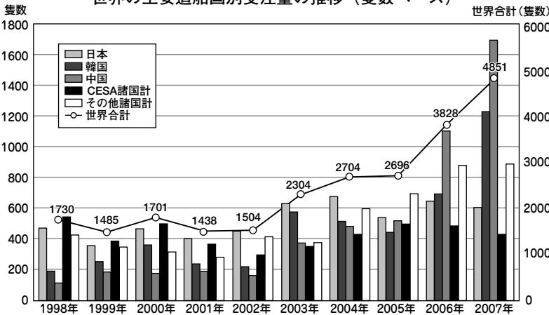
世界の主要造船国別受注量の推移 (隻数ベース)
